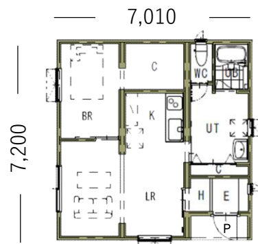
RI-7.2-3型(15.0坪)
