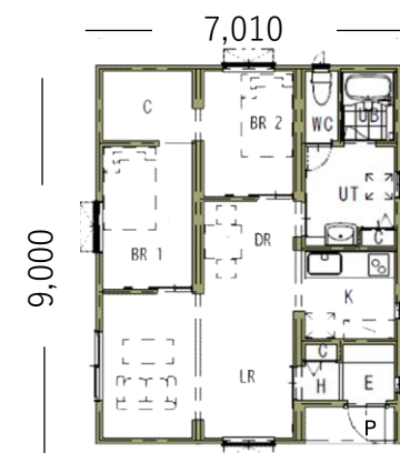
RI-9.0-3型(18.75坪)
