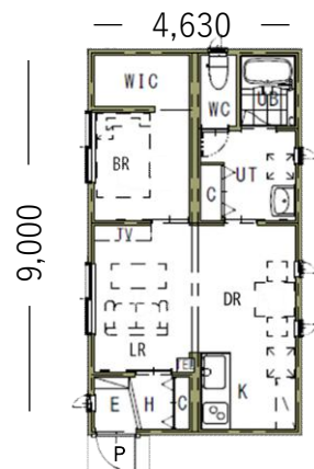
RI-7.2-3型(15.0坪)
