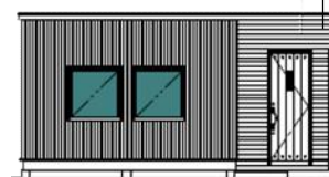
棟側立面図
