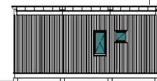
桁側立面図
