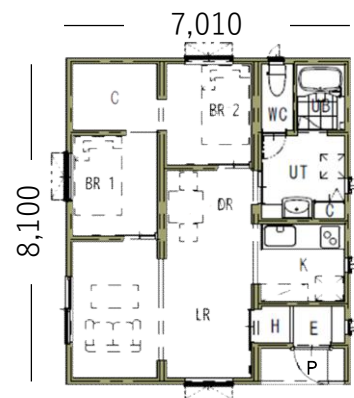
RI-8.1-3型(16.87坪)
